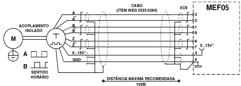
Figura 1.7.1 - Conexão de encoder incremental.
